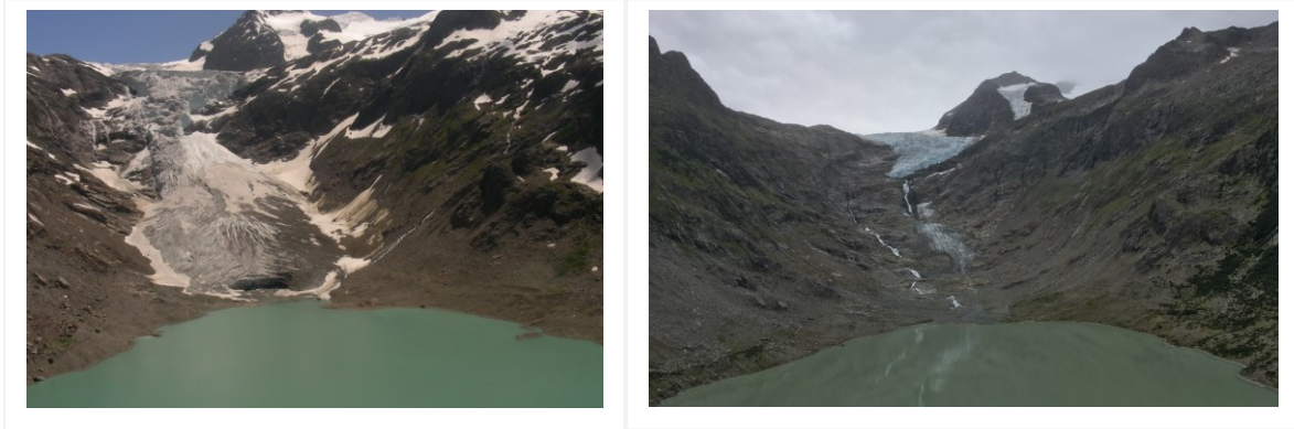
Triftgletscher (Gadmental/BE) 2009 versus 2017 (Fotos: © E. Flükiger)
